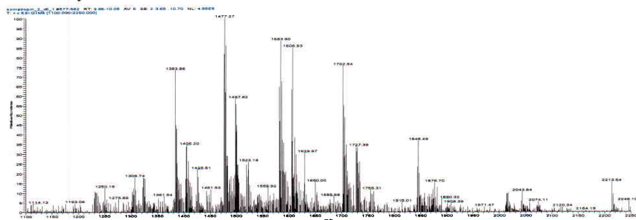
Рисунок 4 – Масс-спектр анализируемого образца, RT = 9,93 мин
