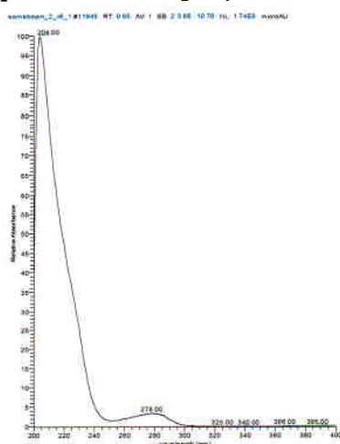
Рисунок 3 – УФ спектр анализируемого образца (диапазон длин волн 190 – 400 нм)
