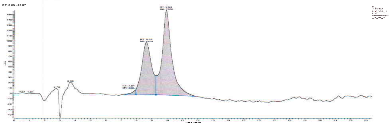
Рисунок 2 – Хроматограмма анализируемого образца 1
